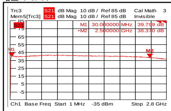
增益 (-45℃)
