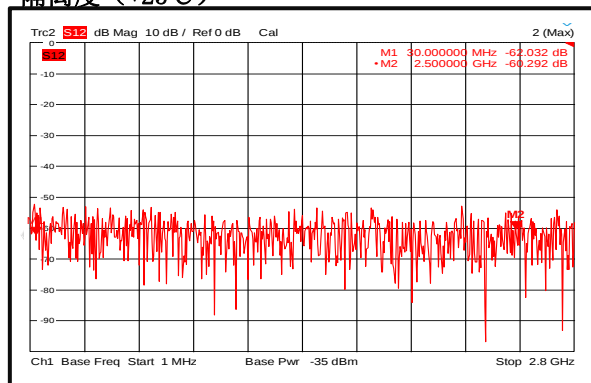
隔离度 (+25℃)
