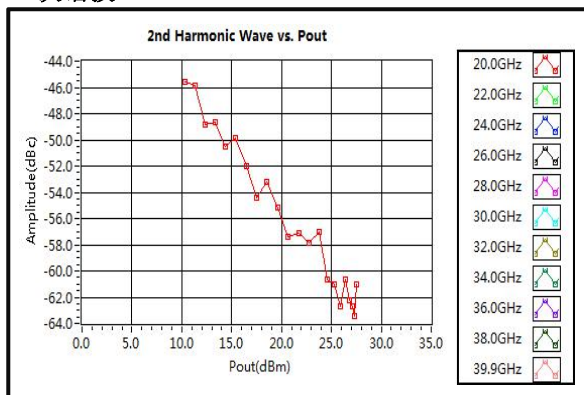
二次谐波
