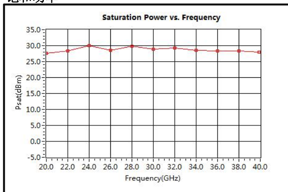
饱和功率
