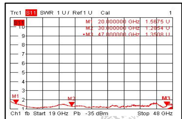
输入驻波比
